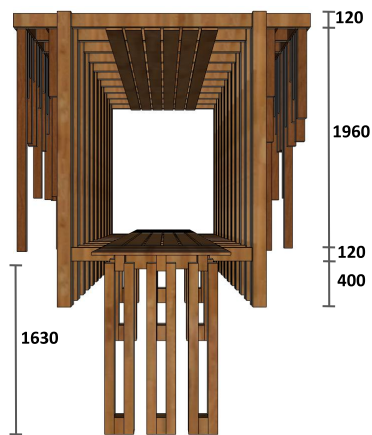
Face Ouest
